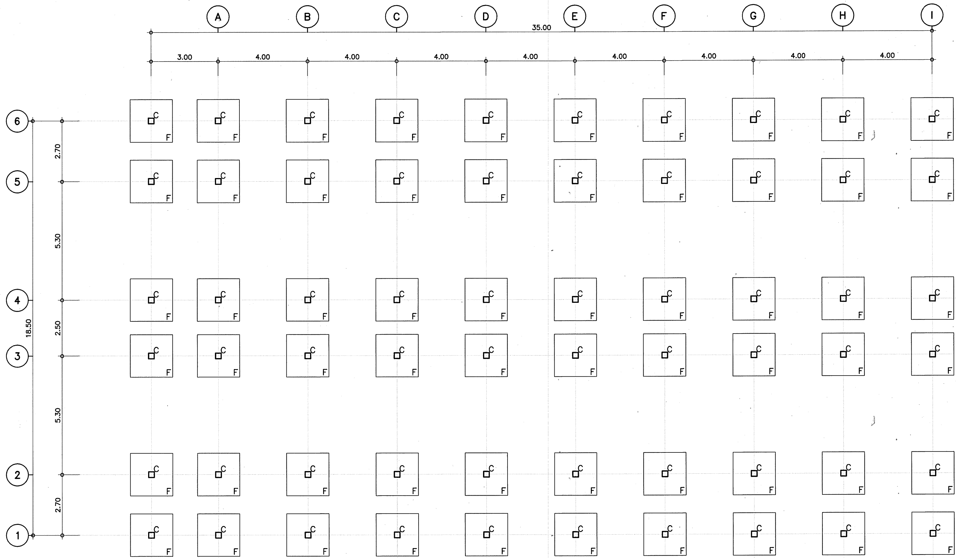
แปลนฐานราก มาตรฐาน 1:100
