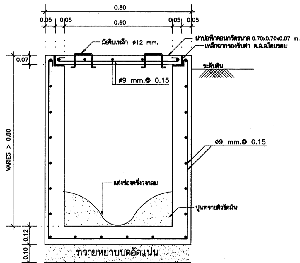
รูปตัด NTS.
