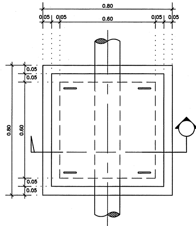
ขยายท่อพักน้ำเลีย (MH.) NTS.
