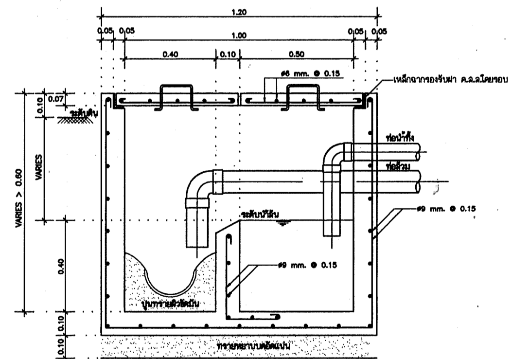
รูปตัด NTS.
