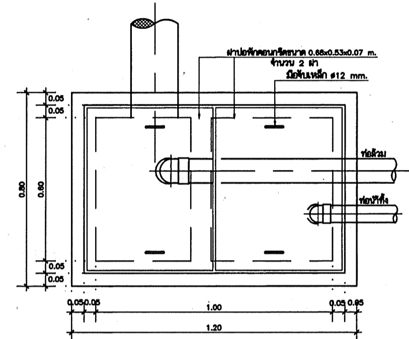
ขยายท่อพักน้ำเลีย NTS.
