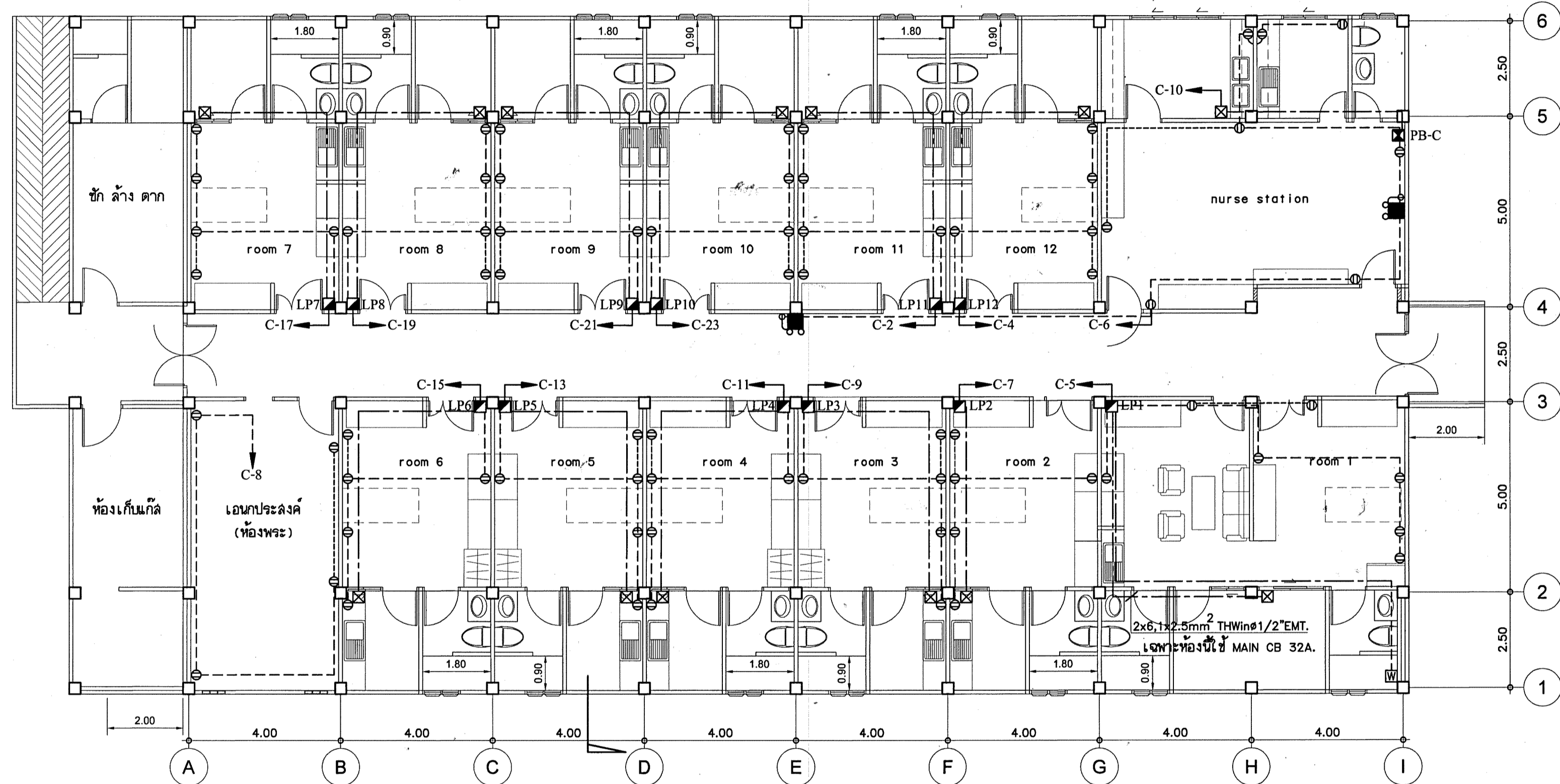
แปลนตัวรับไฟฟ้า มาตรฐาน 1 : 100
