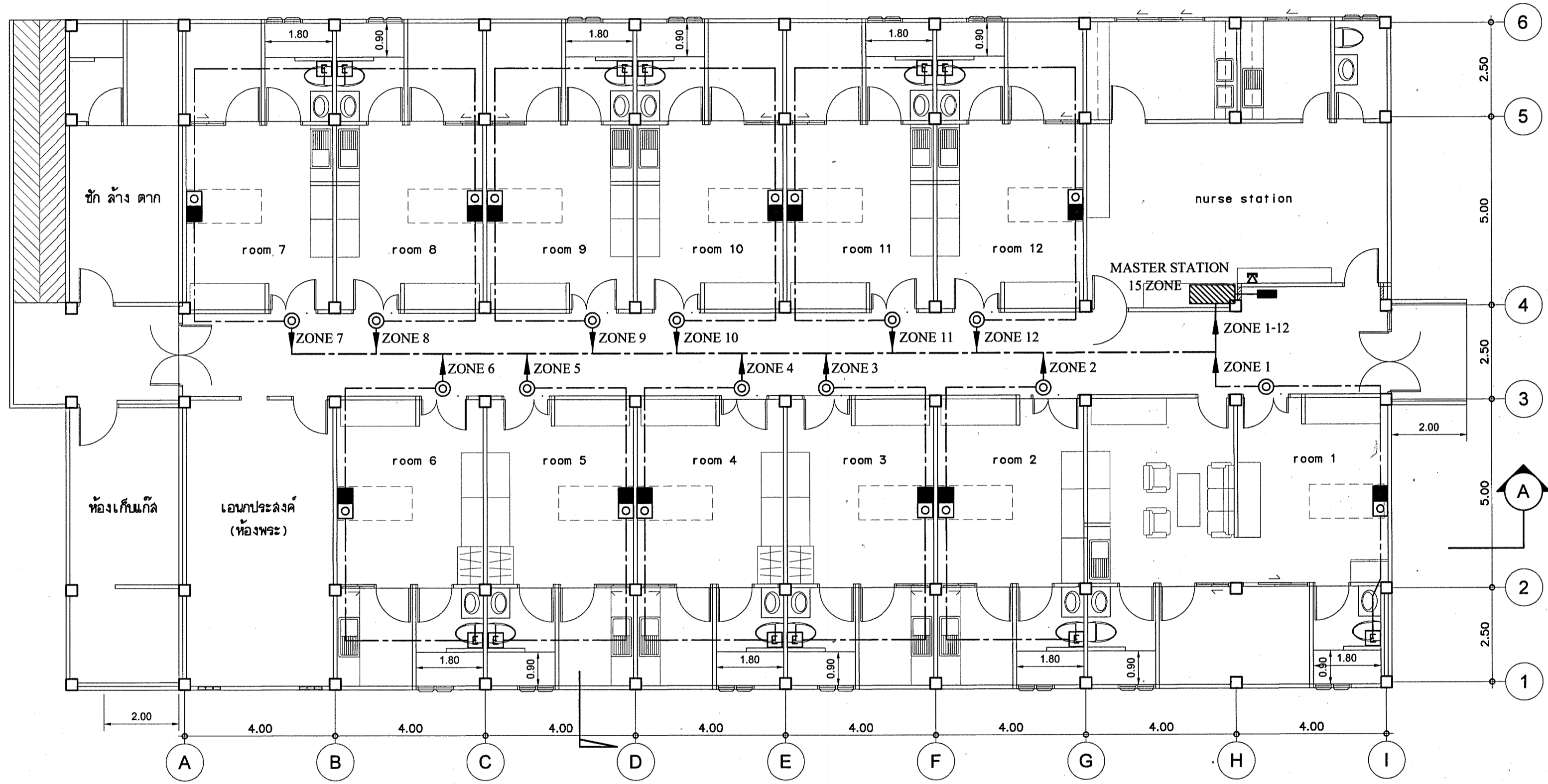
แปลนระบบเรียกพยาบาล มาตรฐาน 1:100
